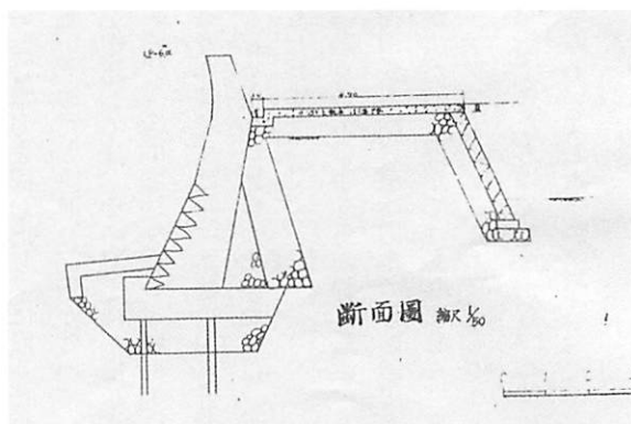
設計図面2 昭和28年の浜戎神社前付近の防潮堤断面図
